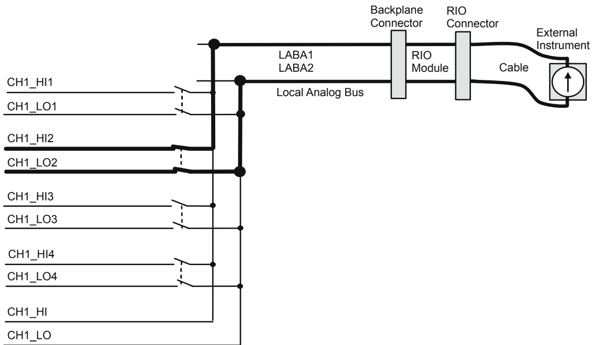
Bild 5-8 Multiplexer - Externe Komponenten, bis 1 A
