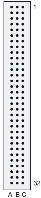
Bild 9-4 R&S TS-PSM2 Steckverbinder X10 (Ansicht: Steckseite)
