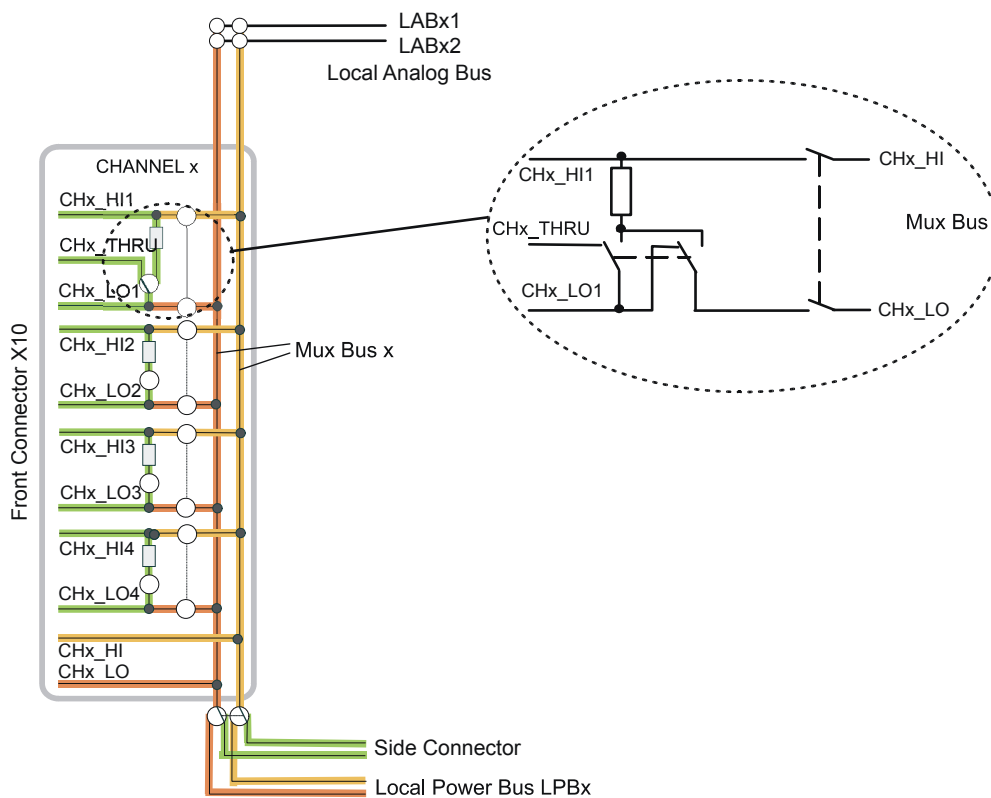
Bild 5-1 Schaltgruppe
