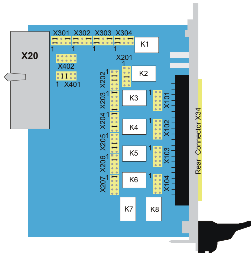
Bild 4-2 Anordnung der Steckverbinder R&S TS-PRIO
