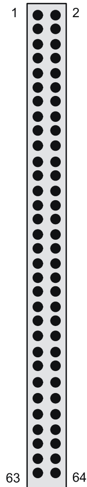
Bild 9-7 R&S TS-PSM2 Steckverbinder X40 (Ansicht: Steckseite)
