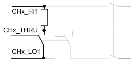
Bild 5-3 Einfache Schaltfunktion - Wechsler, einpolig
