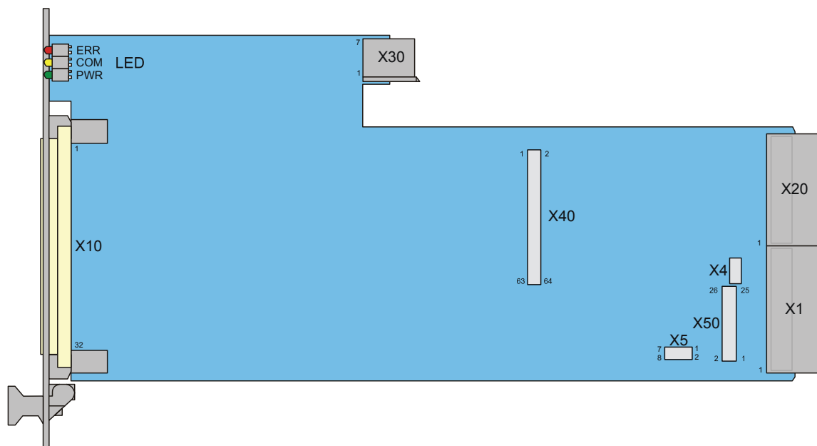
Bild 4-1 Anordnung der Steckverbinder und LEDs R&S TS-PSM2
