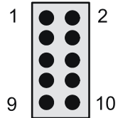
Bild 9-2 R&S TS-PSM2 Steckverbinder X4 (Ansicht: Steckseite)
