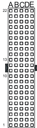
Bild 9-9 R&S TS-PRIO Steckverbinder X20
