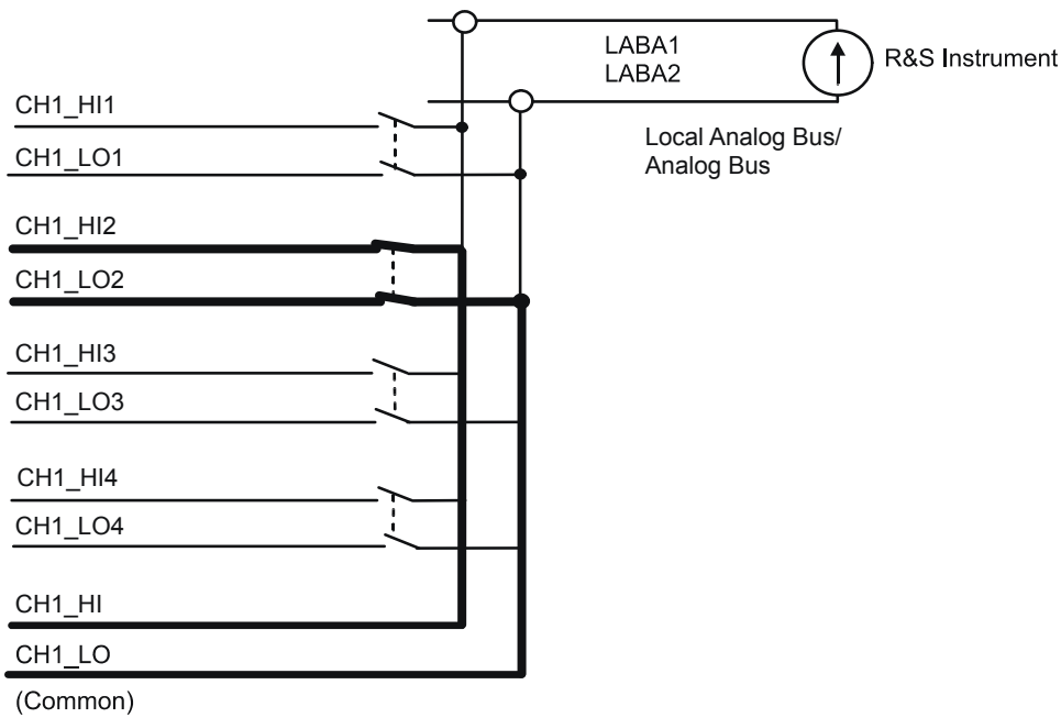
Bild 5-6 Multiplexer - Prüflingssignale
