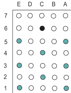
Bild 9-6 R&S TS-PSM2 Steckverbinder X30 (Ansicht: Steckseite)
