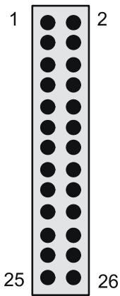
Bild 9-8 R&S TS-PSM2 Steckverbinder X50 (Ansicht: Steckseite)
