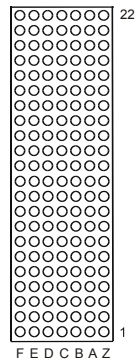
Bild 9-5 R&S TS-PSM2 Steckverbinder X20 (Ansicht: Steckseite)
